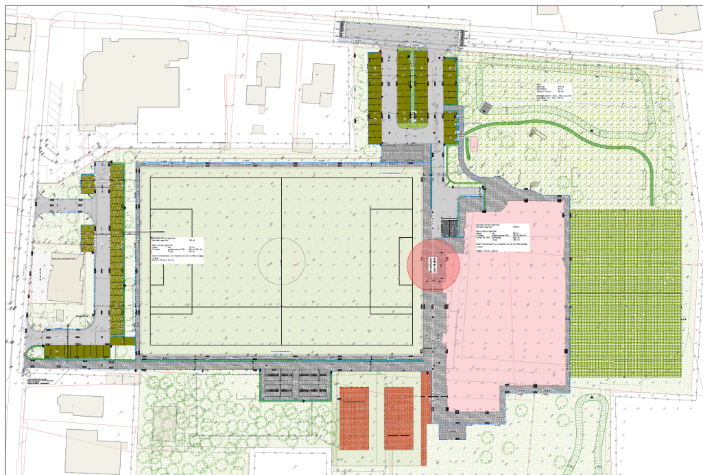
Figuur 5.1 Inrichtingsontwerp buitenruimte MFA Langeveen
