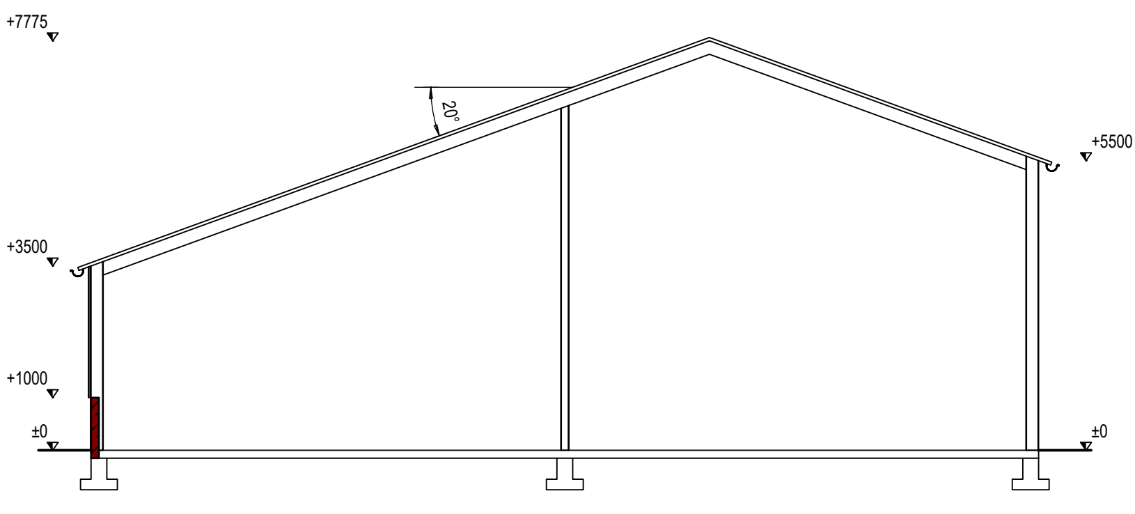
Doorsnede AA
